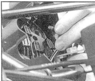
Rimozione lampadina spia Pilot lamp removal Enlèvement de la lampe témoin Herausnahme der Kontrolleuchte
