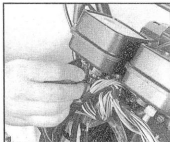
Rimozione lampadina strumento Apparatus bulb removal Enlèvement de l'ampoule de l'instrument Herausnahme der instrumenten-Glühlampe
