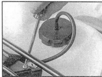
Rimozione supporto spie Removal of the warning lights support Enlèvement du support des témoins Abnehmen der Kontrolleuchten-Fassung
