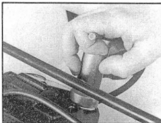
Rimozione ghiera fissaggio interruttore Removal of the ring nut fixing the switch Enlèvement du collier de serrage de l'interrupteur Abschrauben des Gewinderings der Zündschalter-Befestigung
